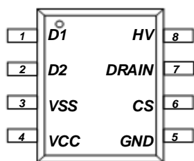
图2 脚位图
