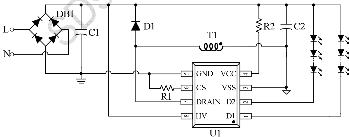
图1 S5533典型应用图
