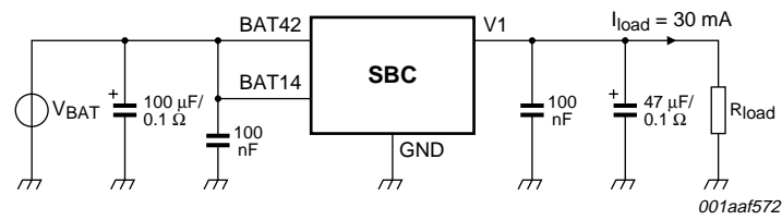
a. Test circuit
